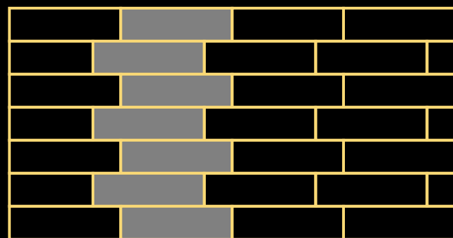
ЛОЖКОВАЯ В ЧЕТВЕРТЬ КИРПИЧА
