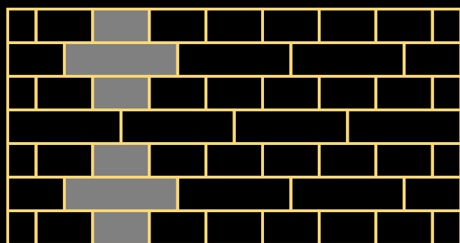
КРЕСТОВАЯ. ТИП II
